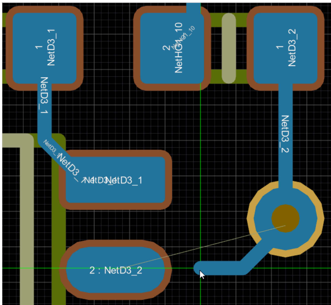
Рисунок 108. Трассировка с переходным отверстием
