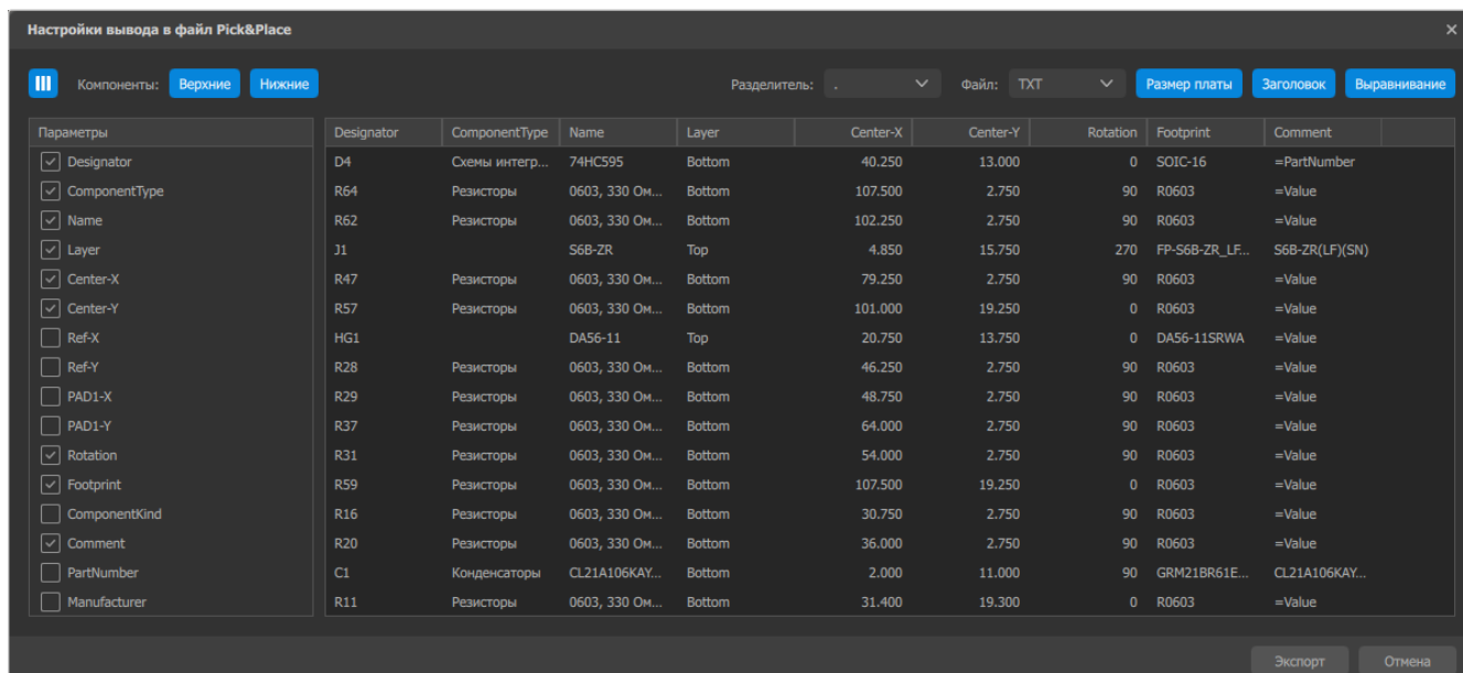
Рисунок 146. Окно «Настройки вывода в файл Pick&Place»
