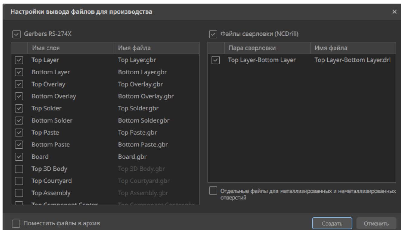
Рисунок 144. Окно «Настройки вывода файлов для производства»
