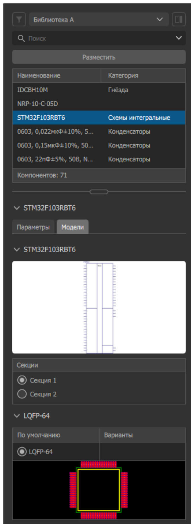
Рисунок 41. Модели компонента в библиотеке компонентов
