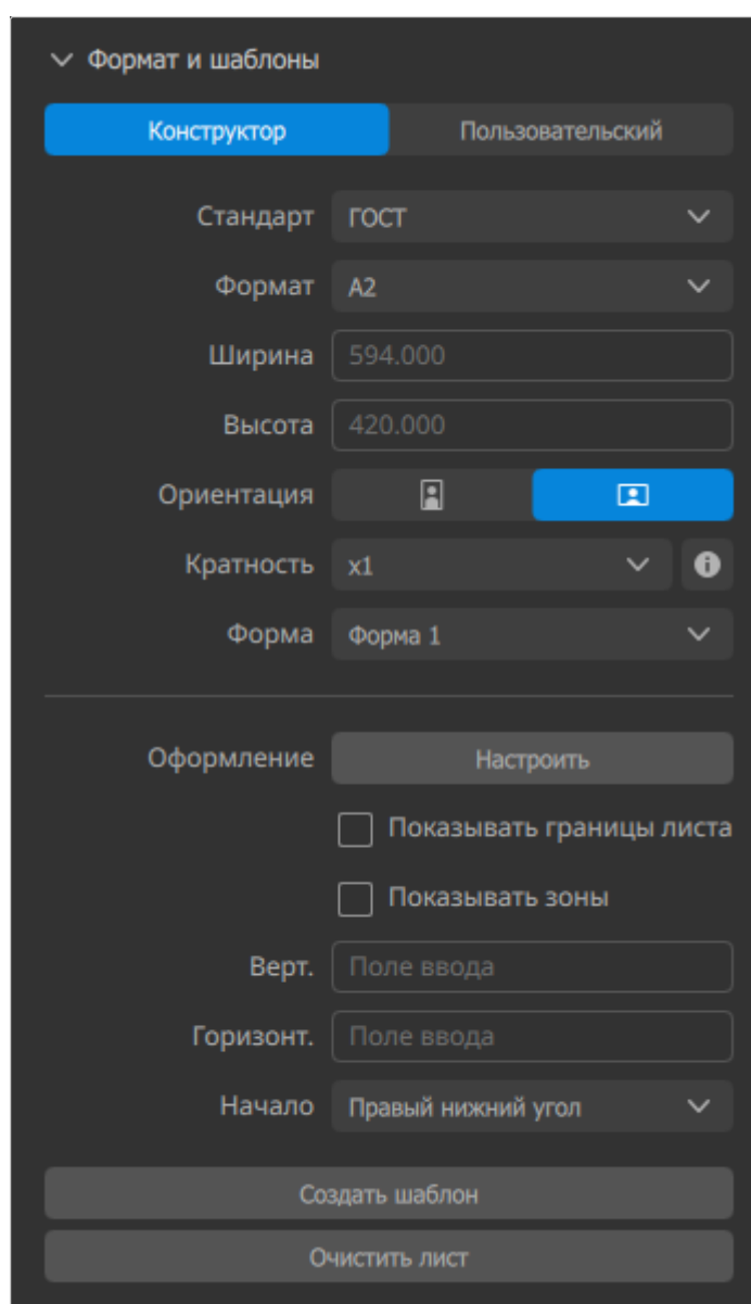
Рисунок 37. Группа «Формат и шаблоны» свойств документа
