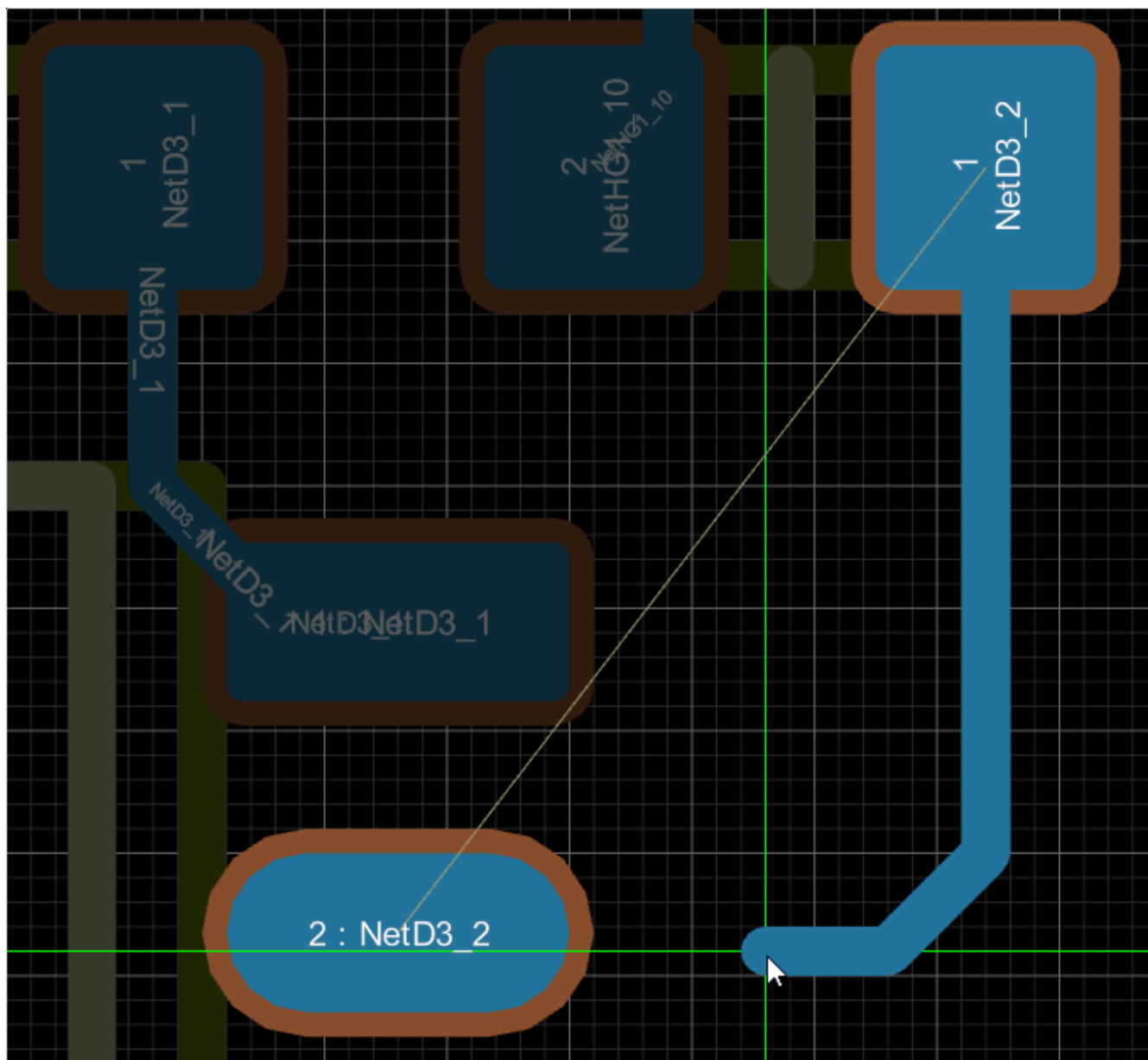
Рисунок 107. Подсветка площадок посадочных мест, объединенных в общую цепь
