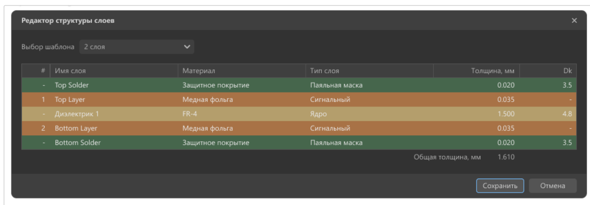
Рисунок 95. Окно «Редактор структуры слоев»
