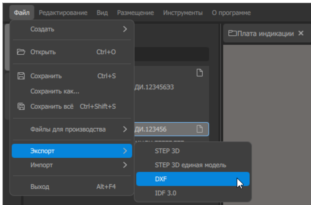
Рисунок 149. Меню «Файл» → Экспорт
